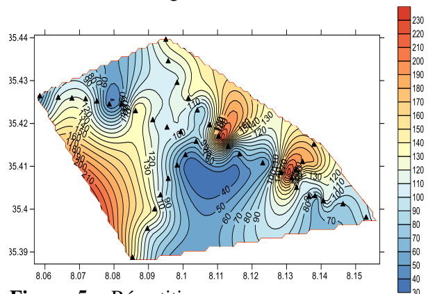
Figure 5 : Répartition de la valeur de bleu de méthylène VBS sur la zone d’étude
