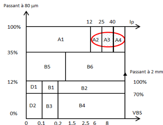
Figure 2 : Classification des matériaux selon leur nature [14]
