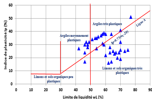
Figure 8 : Classification du sol à base de l'abaque de Casagrande
